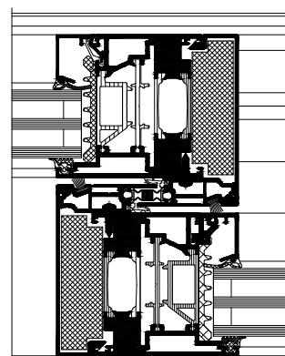
Sezione nodo centrale standard (102 mm)
