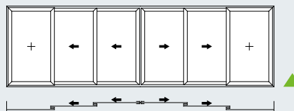
Tipo 3F
